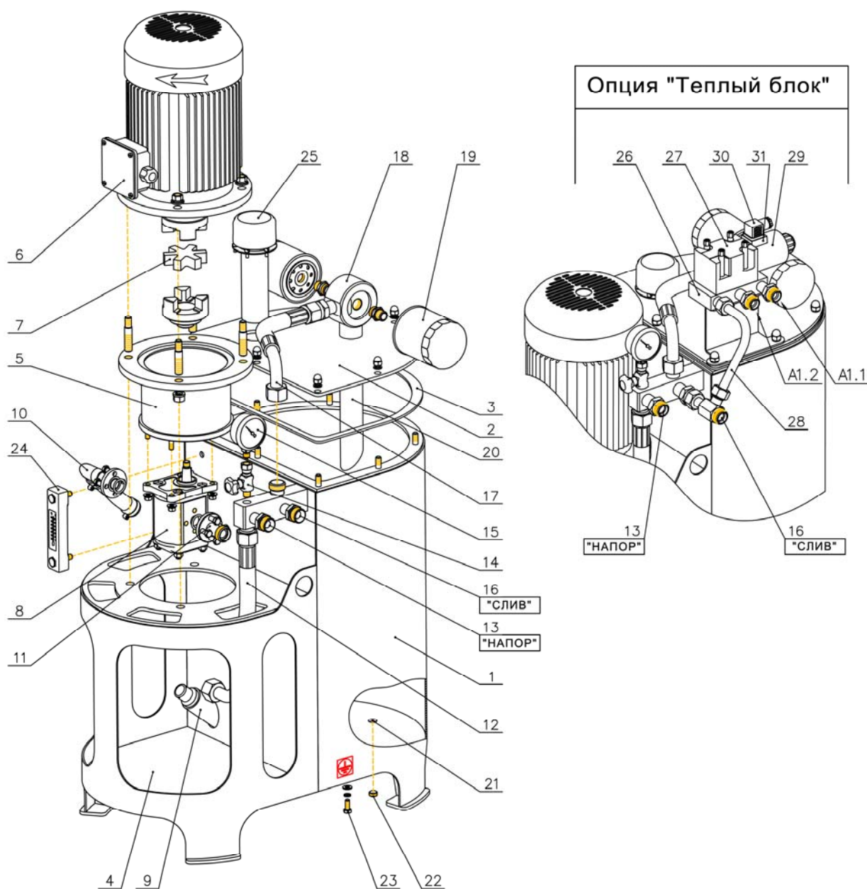
Рис. 5. Установка насосная.
